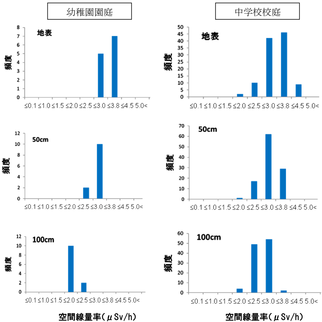
図一 1 福島大学附属中学校校庭及び幼稚園園庭の空間線量率の測定結果 (バックグラウンド未補正)
